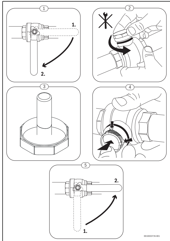
Afb. 5 Filterreiniging
