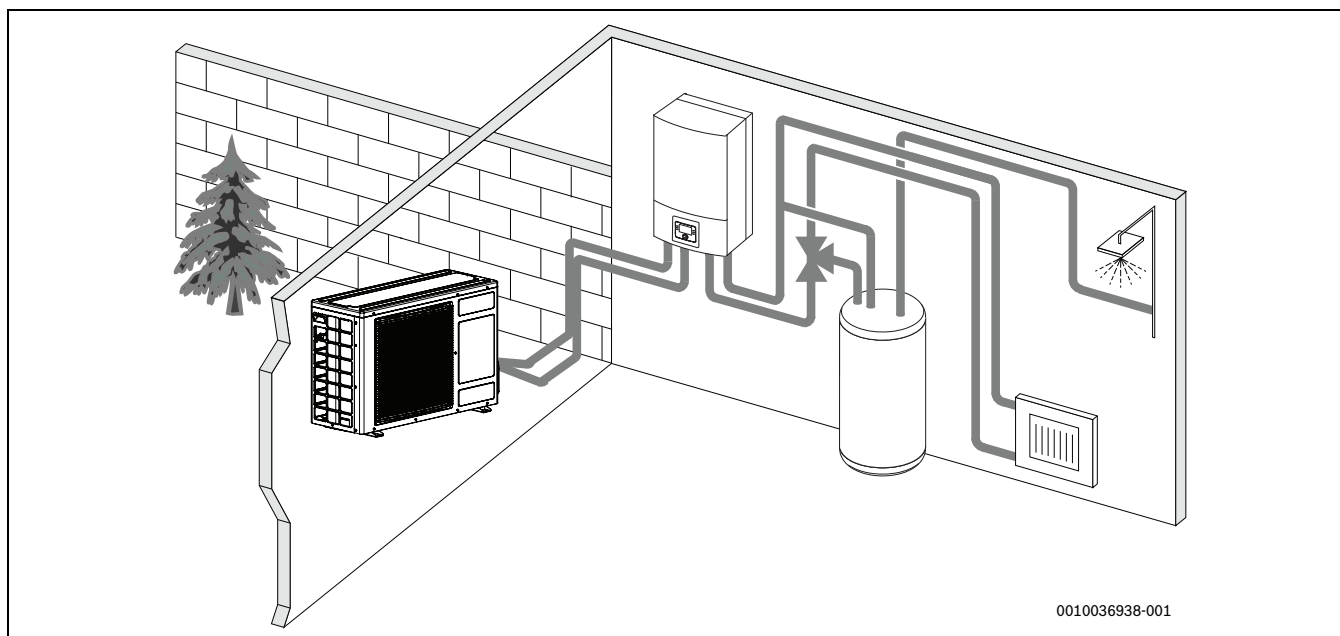
Afb. 2 Warmtepomp buiteneenheid, AWS E binneneenheid met elektrische bijverwarming en externe boiler
