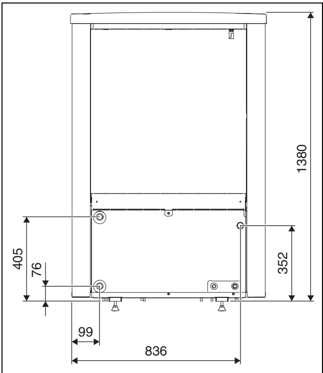
Fig. 4 Dimensions et raccords des modèles de pompe à chaleur 5 OR-7 OR, partie arrière
