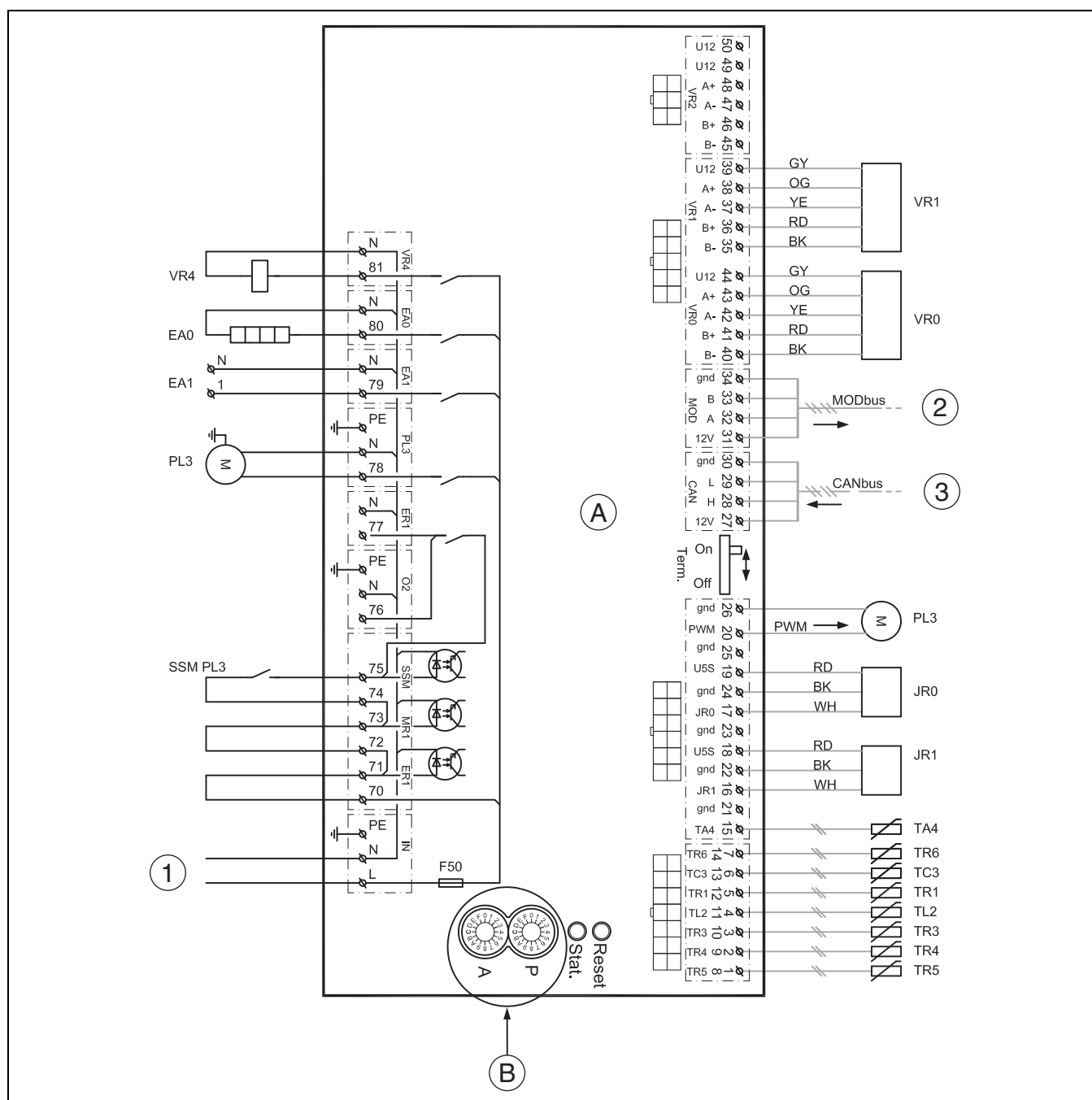
Fig. 22 Schéma de connexion pour module I/O
