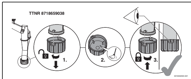
Fig. 64 Nettoyer le filtre.
