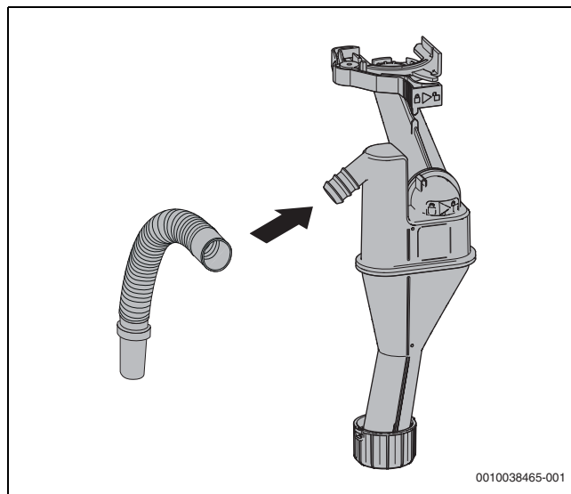
Fig. 33 Placer l'évacuation des condensats sur le raccord
