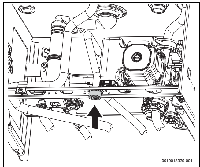
Bild 22 Anschluss externes Ausdehnungsgefäß
