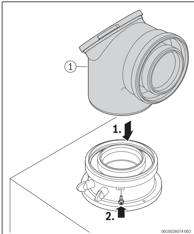
Bild 29 Abgaszubehör einsetzen und mit Schraube sichern
