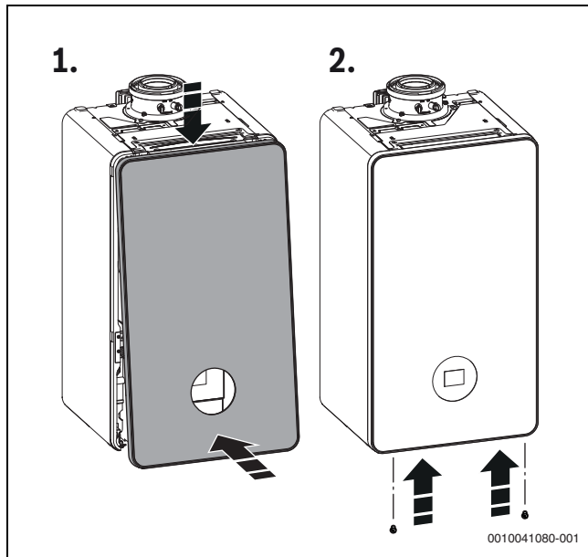
Bild 34 Verkleidung montieren
