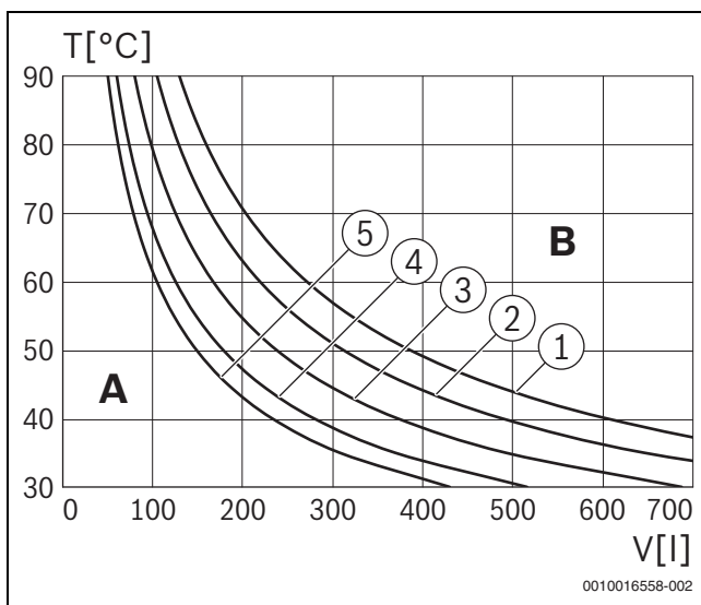
Bild 23 Kennlinien des Ausdehnungsgefäßes
