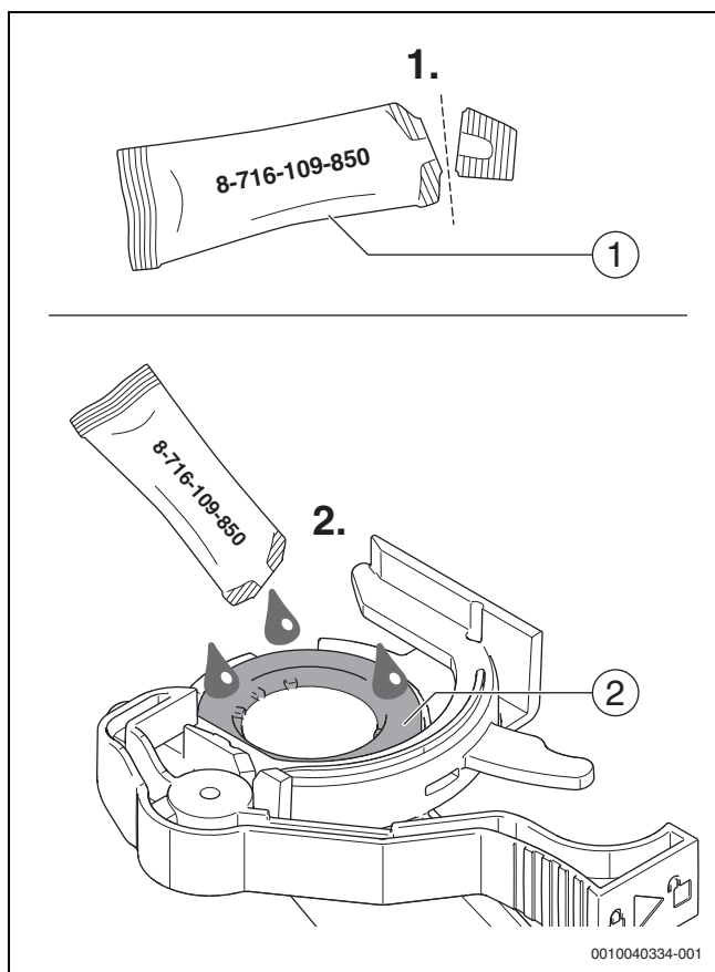
Bild 55 Dichtung fetten
