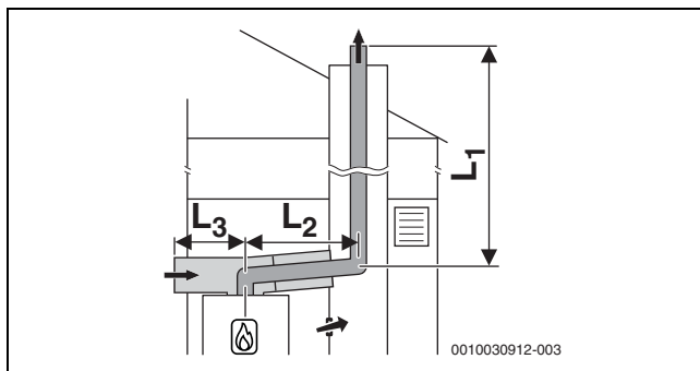
Bild 12 Starre Abgasführung nach C 53x im Schacht und Luft-Abgas-Führung mit separater Luftzufuhr und konzentrischer Abgasleitung im Aufstellraum
