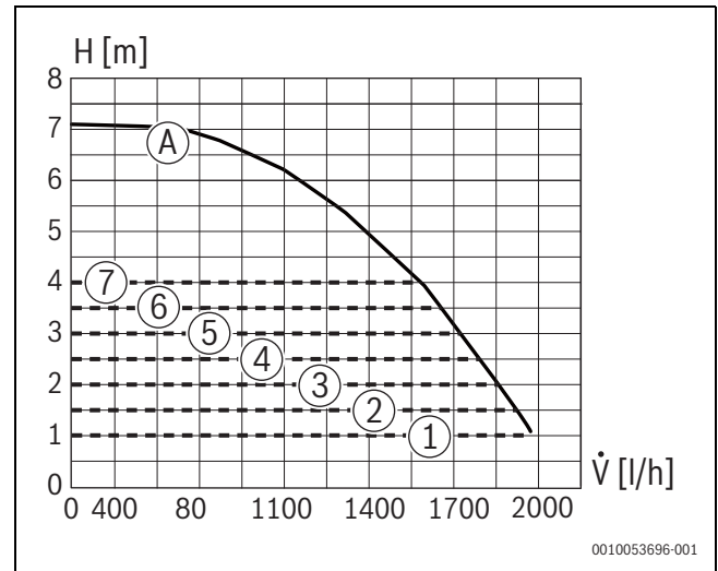
Bild 63 Pumpenkennfelder und Pumpenkennlinien GC7700iW 45 P 23
