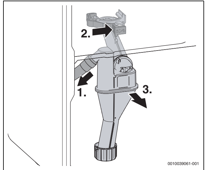
Bild 52 Kondensatsiphon ausbauen
