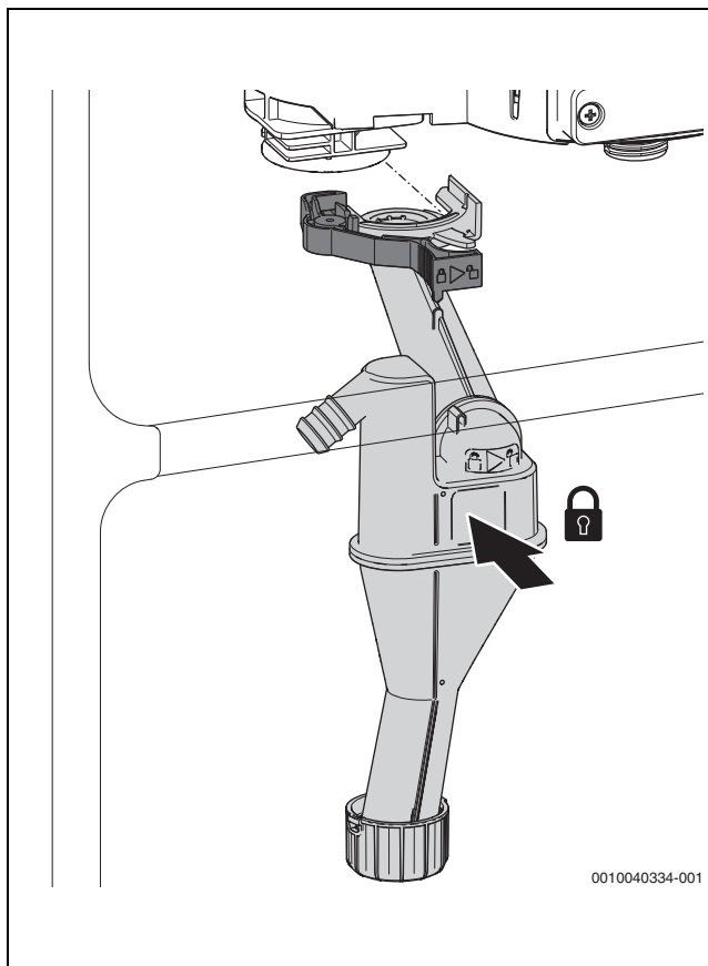
Bild 56 Kondensatsiphon einsetzen
