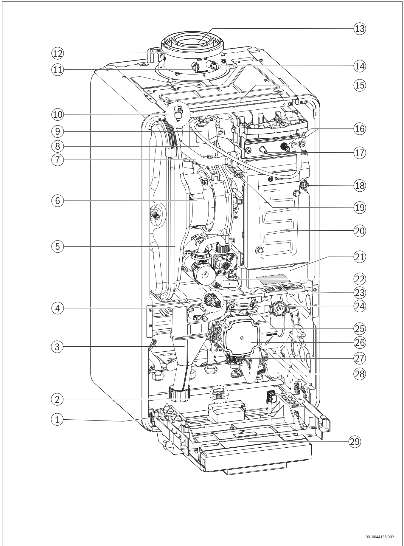
Bild 5 Produktübersicht Speichergerät
