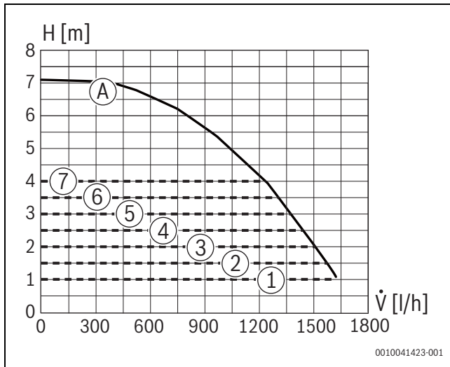
Bild 61 Pumpenkennfelder und Pumpenkennlinien GC7700iW 30/35 C 23, GC7700iW 30/50 C 23, GC7700iW 30/35 C 31, GC7700iW 30/50 C 31
