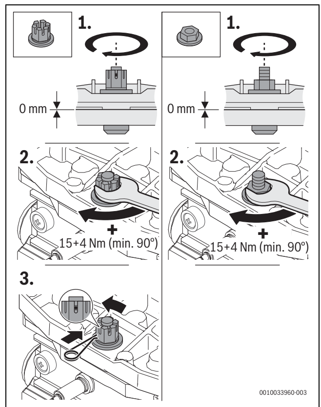
Bild 45 Mutter am Brennerdeckel festziehen
