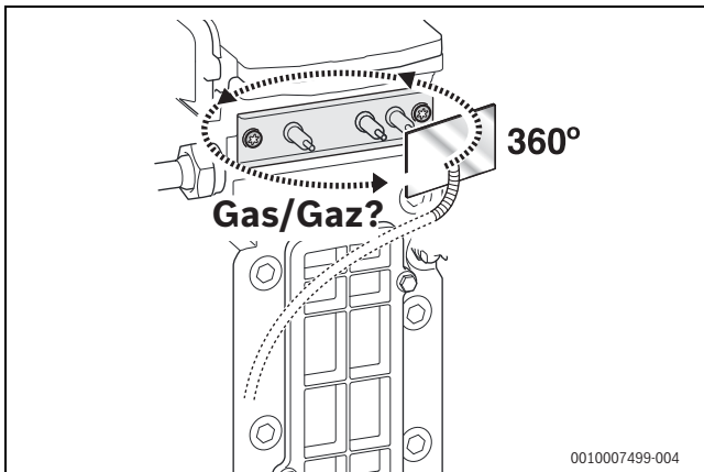
Bild 42 Dichtigkeit prüfen
