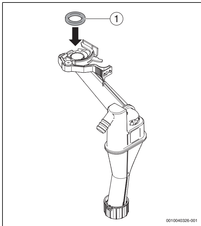
Bild 54 Neue Dichtung am Kondensatsiphon einsetzen
