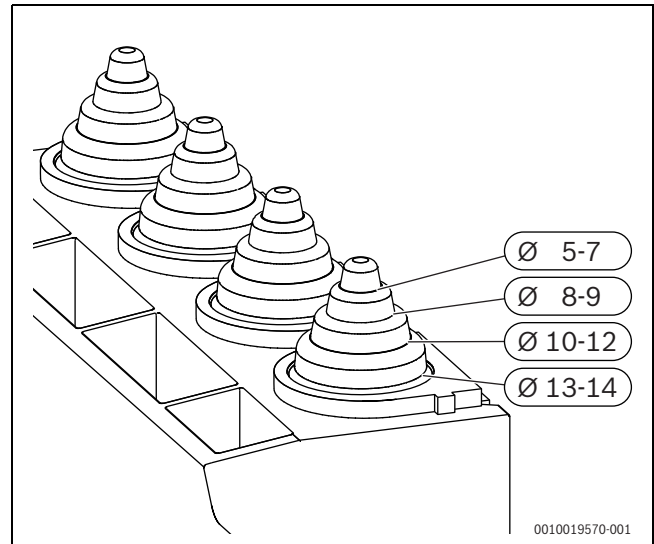
Bild 32 Zugentlastung an Kabeldurchmesser anpassen
