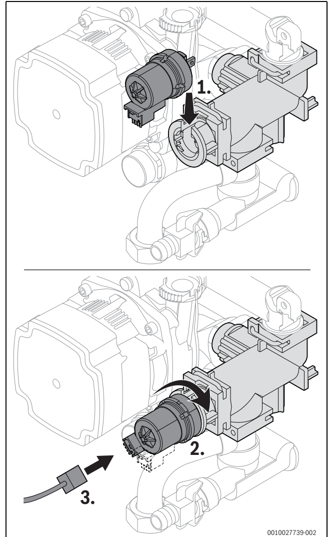
Bild 58 Motor am 3-Wege-Ventil einbauen (Variante ohne Schrauben)
