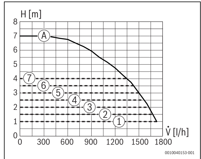
Bild 62 Pumpenkennfelder und Pumpenkennlinien GC7700iW 35 P 23, GC7700iW 35 P 31
