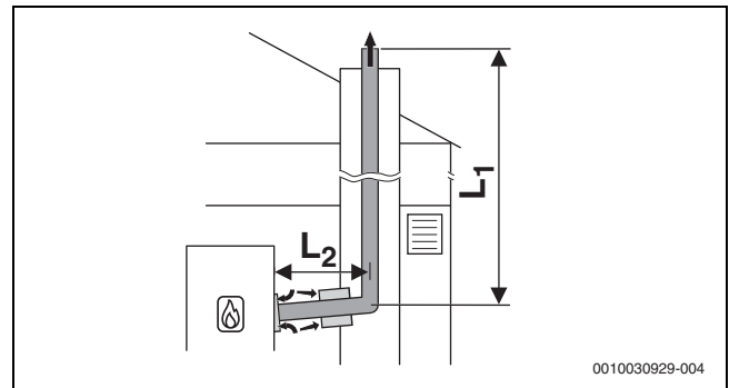
Bild 17 Starre Abgasführung im Schacht nach B 23p mit raumluftabhängiger Luftzufuhr am Gerät und konzentrischem Verbindungsstück zwischen Aufstellraum und Schacht
