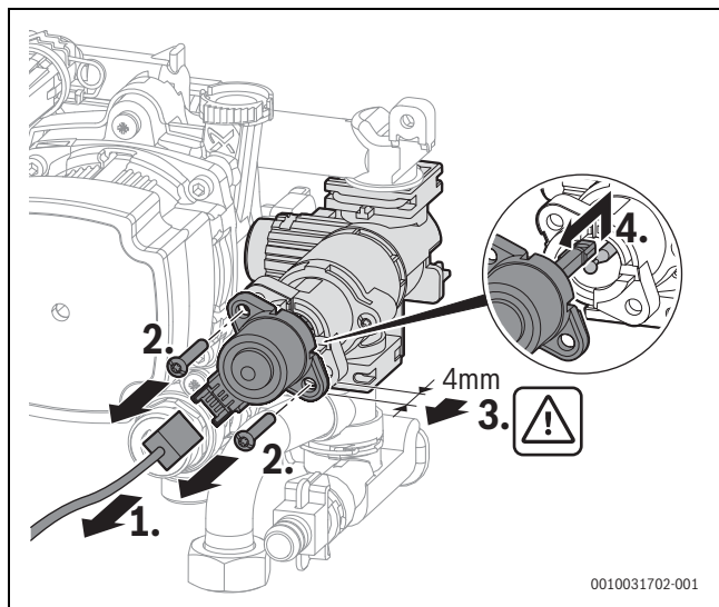
Bild 59 Motor am 3-Wege-Ventil ausbauen (Variante mit Schrauben)
