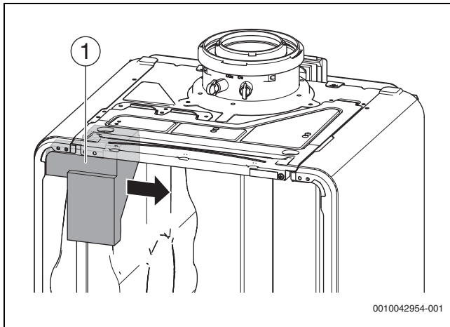
Bild 25 Stützschaum entfernen
