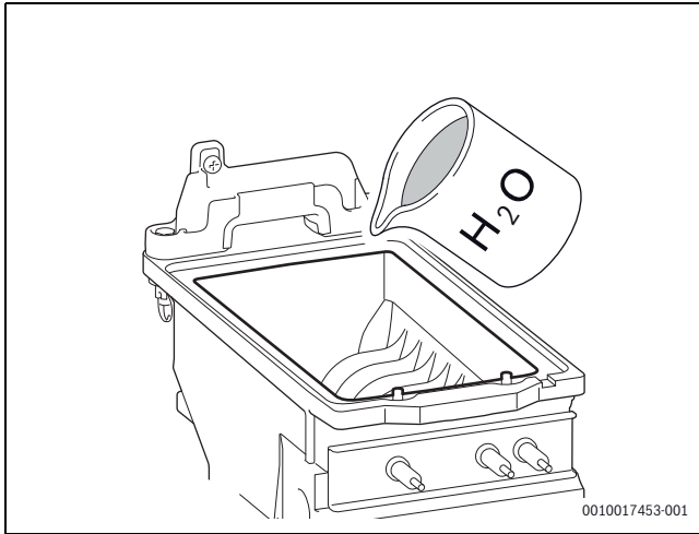
Bild 50 Wärmeblock spülen
