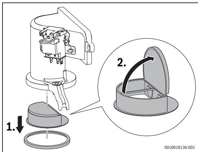
Bild 47 Rückschlagklappe in der Mischeinrichtung
