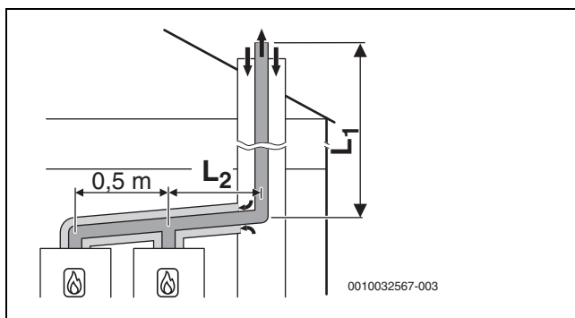
Bild 20 Kaskade mit 2 Geräten: Starre Abgasführung nach C 93x im Schacht und konzentrische Luft-Abgas-Führung im Aufstellraum
