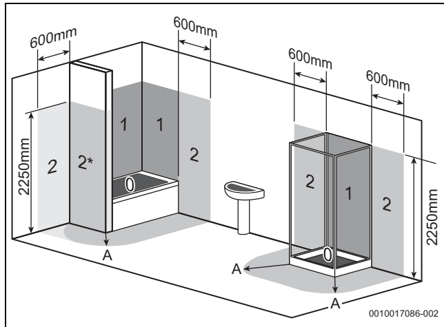
Bild 21 Schutzbereiche (Beispieldarstellung)
