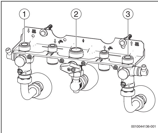
Bild 30 Gas- und wasserseitige Anschlüsse
