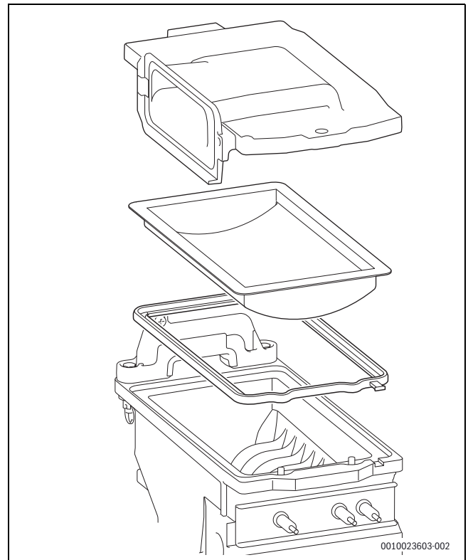
Bild 44 Brenner
