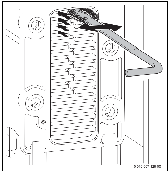
Bild 49 Wärmeblock mit Bürste reinigen
