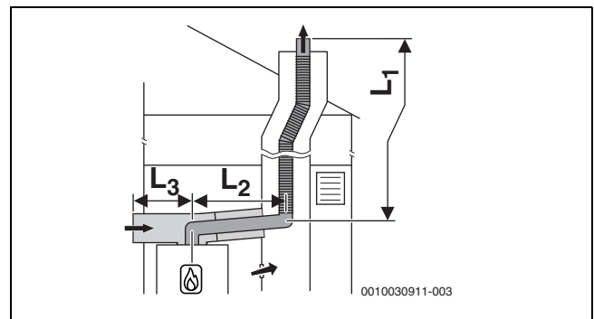
Bild 13 Flexible Abgasführung nach C 53x im Schacht und Luft-Abgas-Führung mit separater Luftzufuhr und konzentrischer Abgasleitung im Aufstellraum
