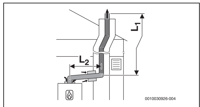
Bild 18 Flexible Abgasführung im Schacht nach B 23p mit raumluftabhängiger Luftzufuhr am Gerät und konzentrischem Verbindungsstück zwischen Aufstellraum und Schacht
