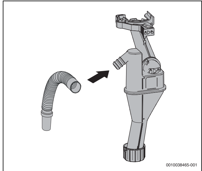
Bild 27 Kondensatablauf auf das Anschlussstück stecken
