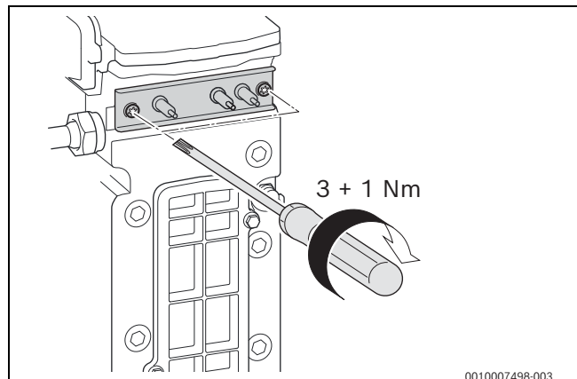
Bild 41 Elektroden-Set montieren
