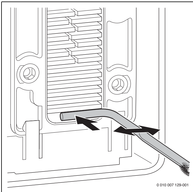
Bild 51 Kondensatwanne reinigen
