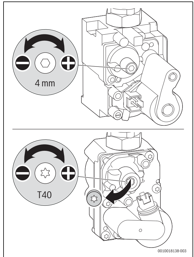
Bild 38 CO 2 - oder O 2 -Gehalt einstellen
