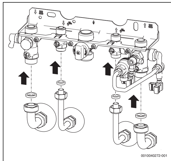
Bild 24 Rohre mit Dichtungen an Montageanschlussplatte montieren
