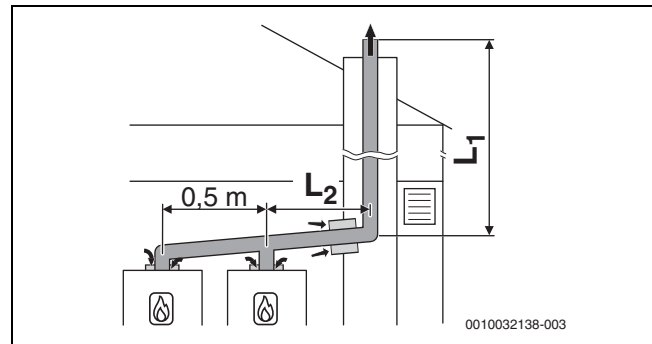
Bild 19 Kaskade mit 2 Geräten: Starre Abgasführung im Schacht nach B 53p mit raumluftabhängiger Luftzufuhr am Gerät
