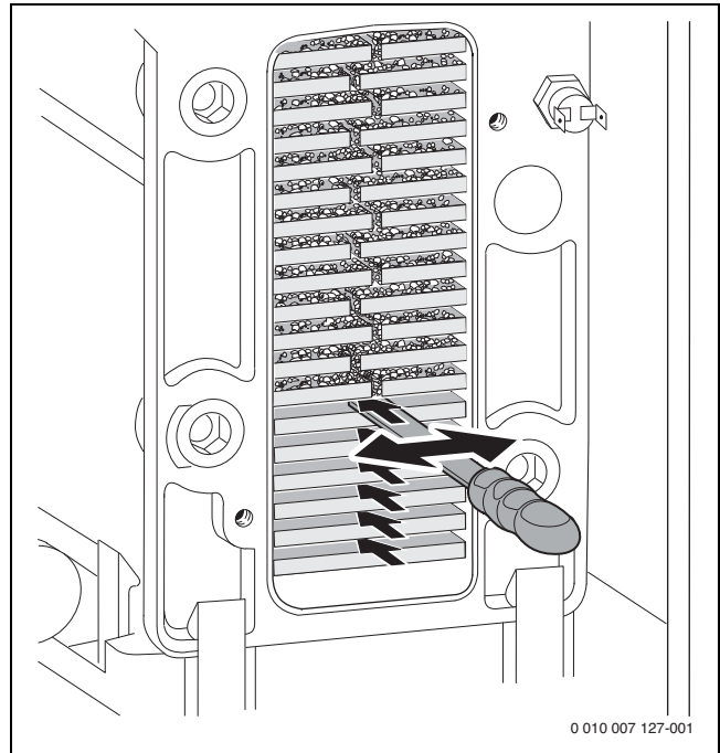
Bild 48 Reinigungsmesser
