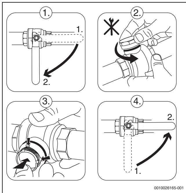
Fig. 32 Montage et démontage du filtre de particules (exemple)
