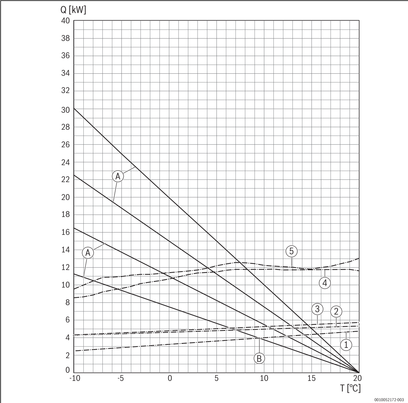
Fig. 31 Diagramme du tableau 9 ; pour déterminer les points de bivalence de la température pour une température de départ de 65 °C
