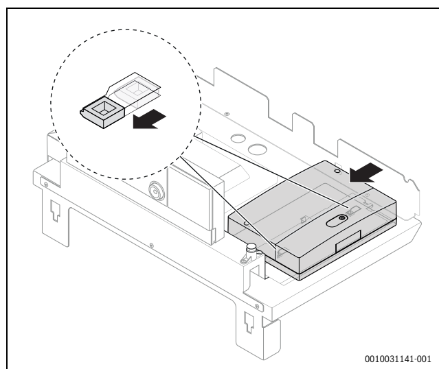
Fig. 18 Montage du module électronique sous le capot de la chaudière (exemple)
