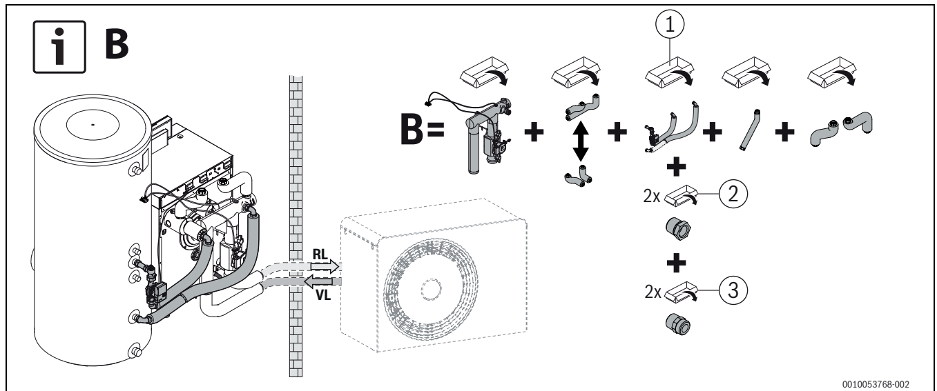
Fig. 13 Connexion ballon vertical à droite, variante B, exemple d'illustration pour taille de chaudière 15 kW
