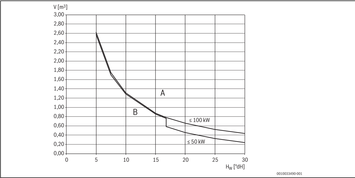
Fig. 24 Limites du traitement de l'eau
