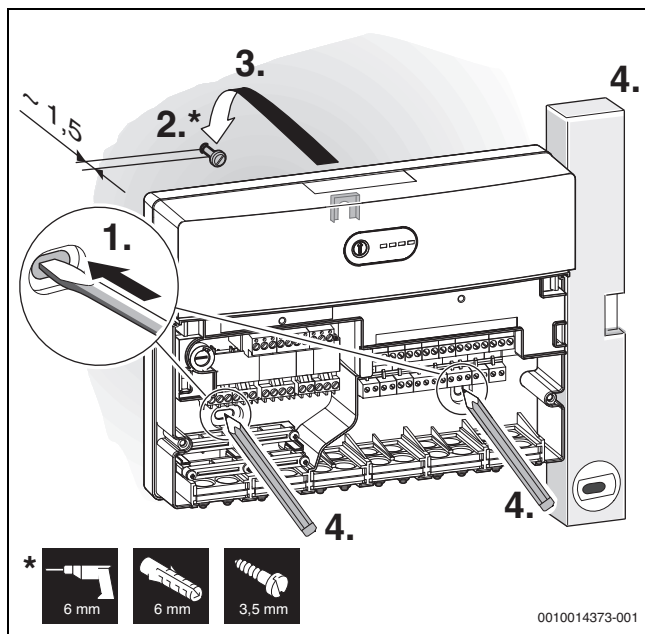
Fig. 21 Marquer la fixation murale
