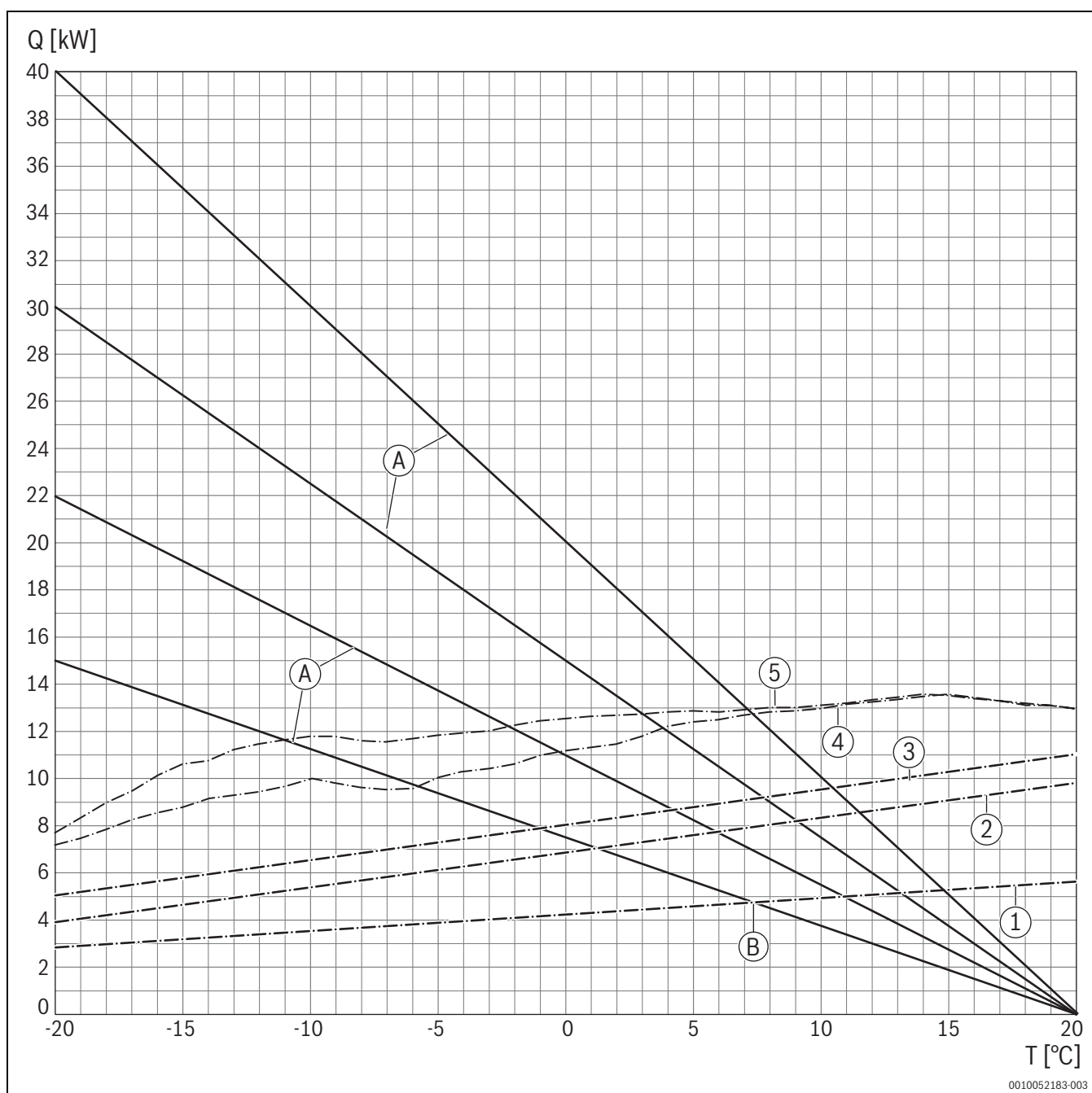
Fig. 26 Diagramme du tableau 4 ; pour déterminer les points de bivalence de la température pour une température de départ de 35 °C
