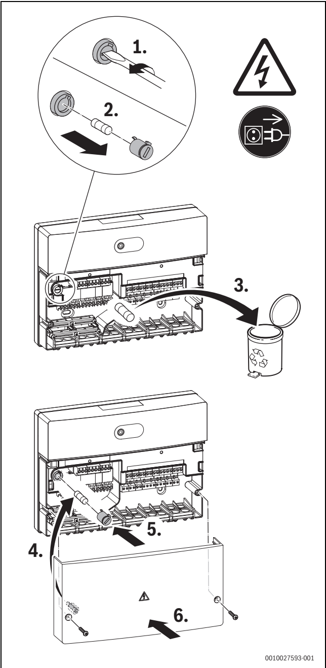
Fig. 34 Remplacer le fusible
