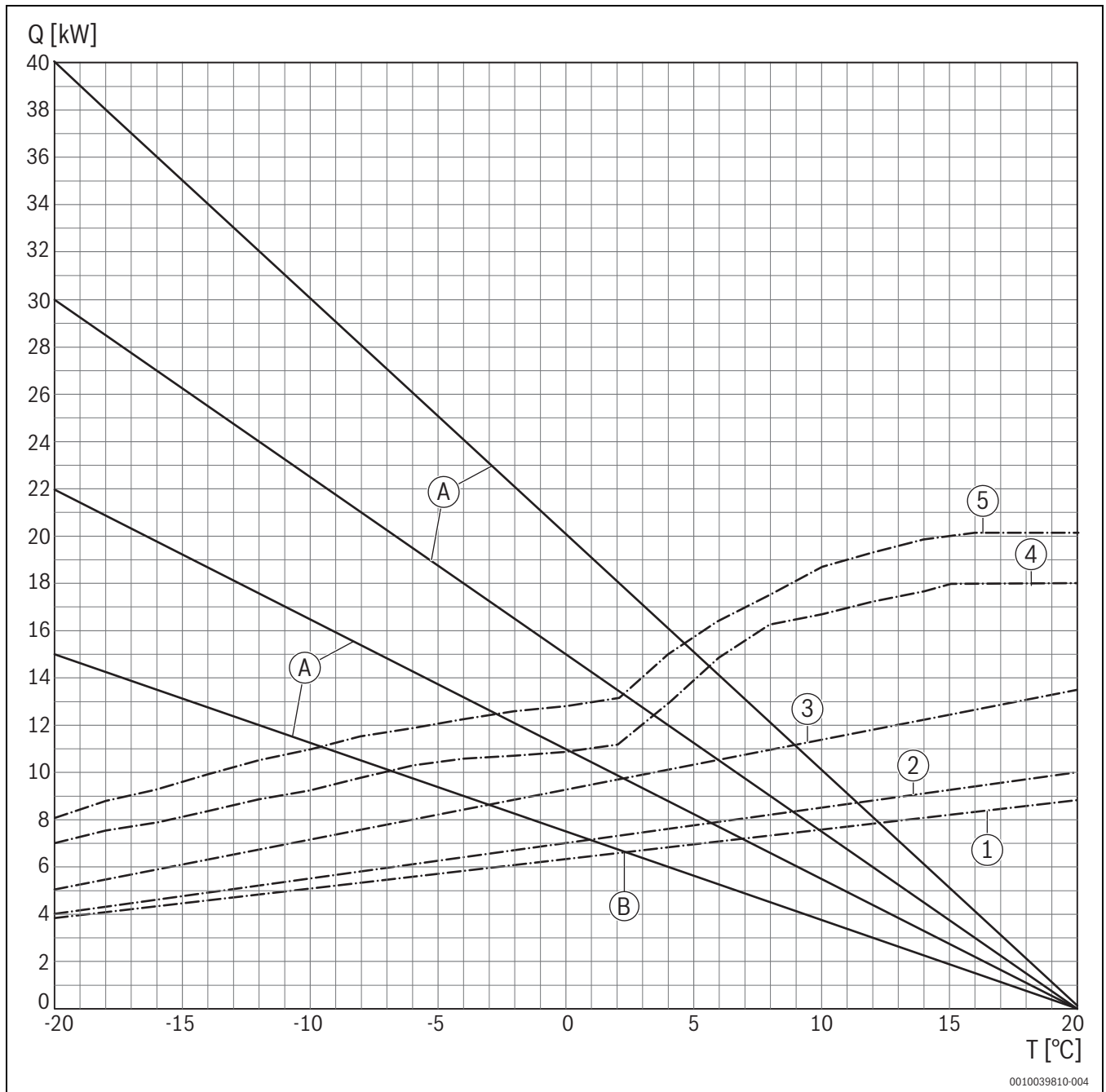
Fig. 27 Diagramme du tableau 5 ; pour déterminer les points de bivalence de la température pour une température de départ de 45 °C
