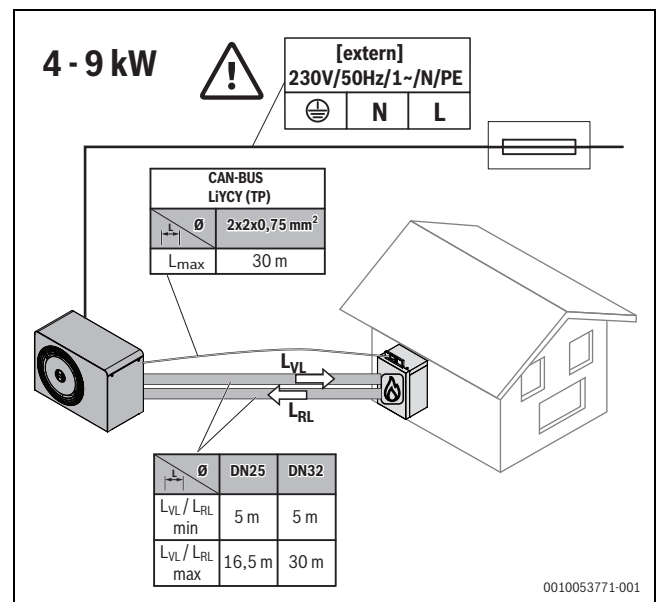
Fig. 8 Exigences relatives à la longueur des conduites 4 – 9 kW
