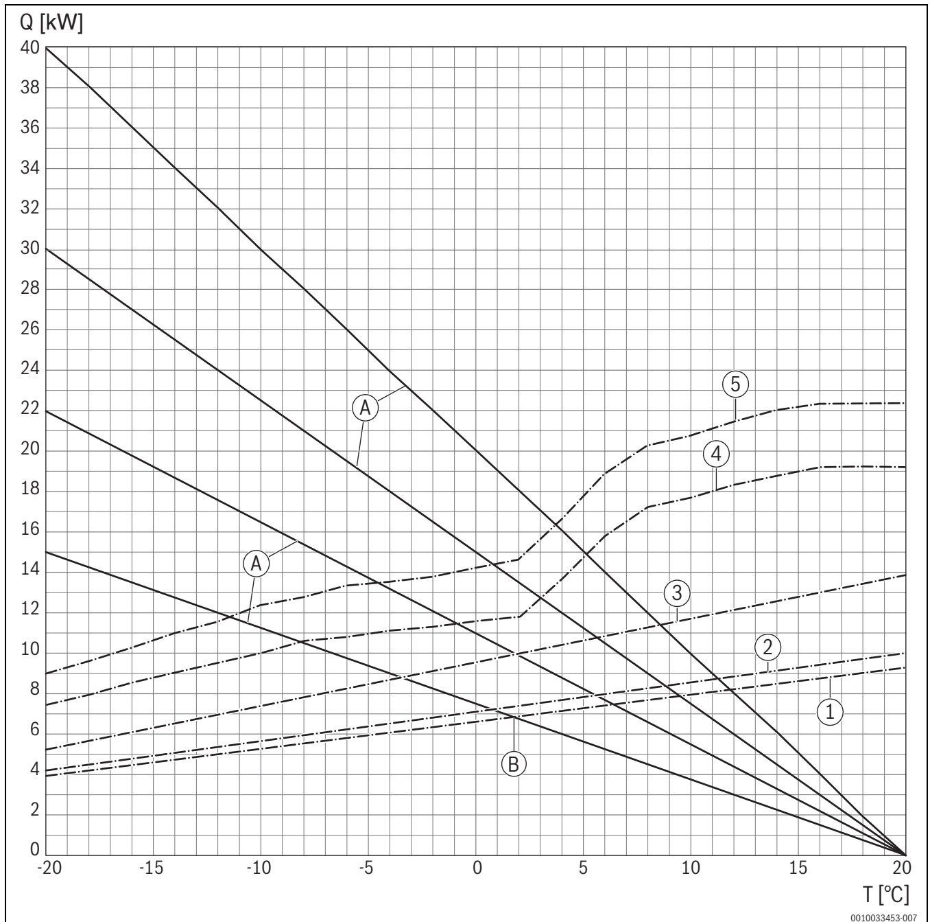
Fig. 25 Diagramme du tableau 3 ; pour déterminer les points de bivalence de la température pour une température de départ de 35 °C
