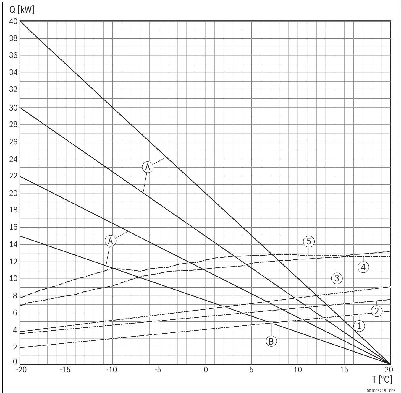
Fig. 30 Diagramme du tableau 8 ; pour déterminer les points de bivalence de la température pour une température de départ de 55 °C
