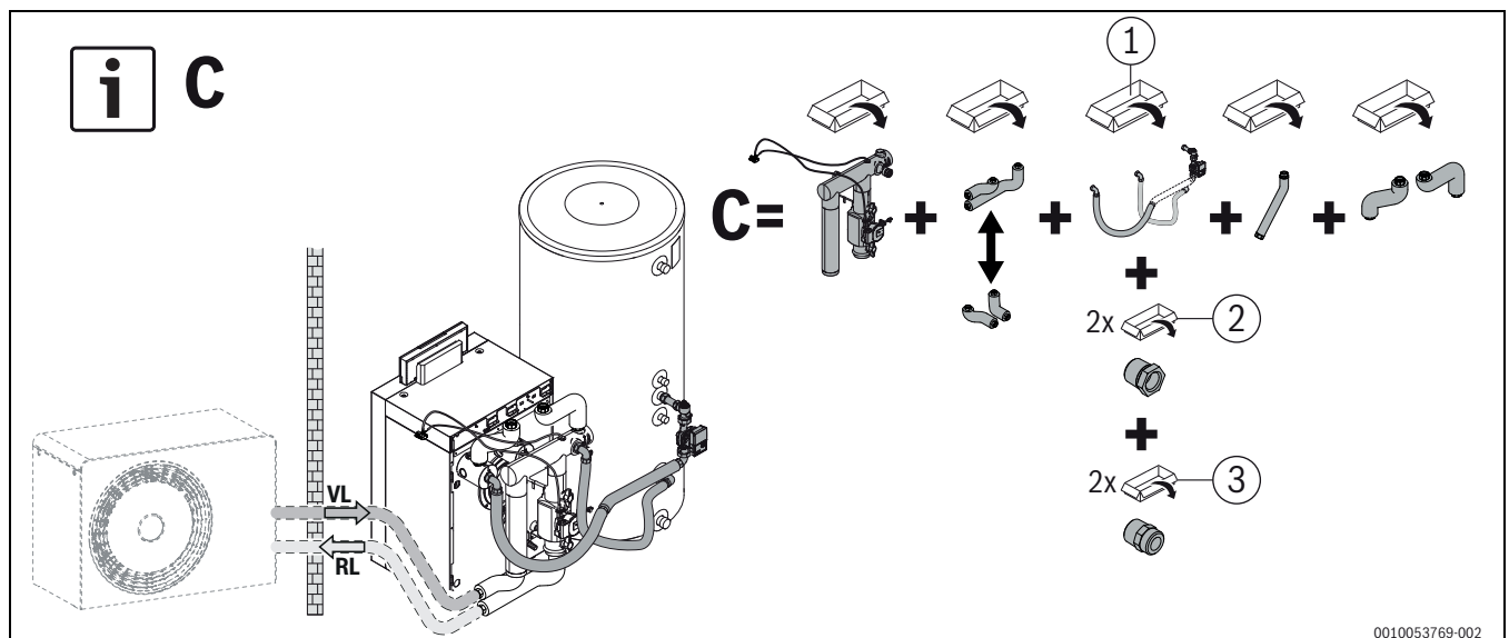
Fig. 14 Connexion ballon vertical à gauche, variante C, exemple d'illustration pour taille de chaudière 15 kW
