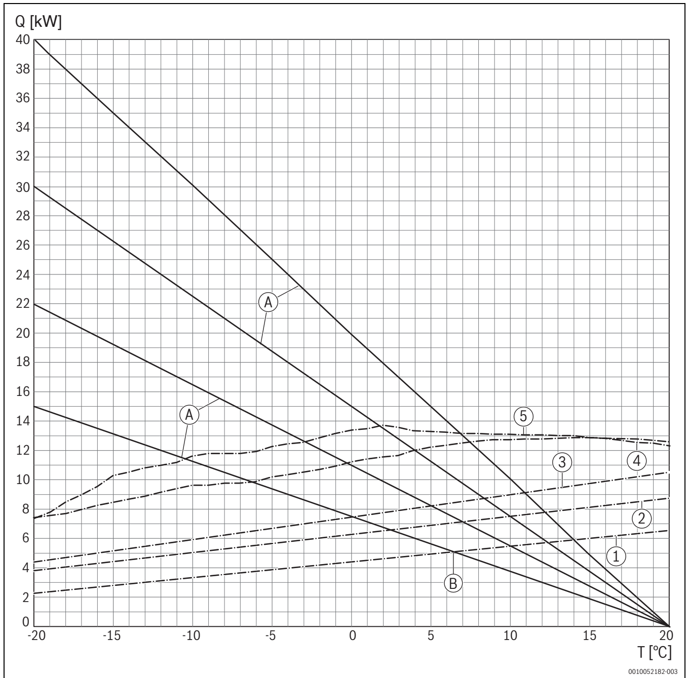
Fig. 28 Diagramme du tableau 6 ; pour déterminer les points de bivalence de la température pour une température de départ de 45 °C
