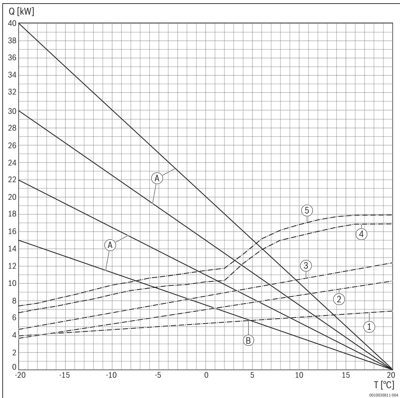
Fig. 29 Diagramme du tableau 7 ; pour déterminer les points de bivalence de la température pour une température de départ de 55 °C
