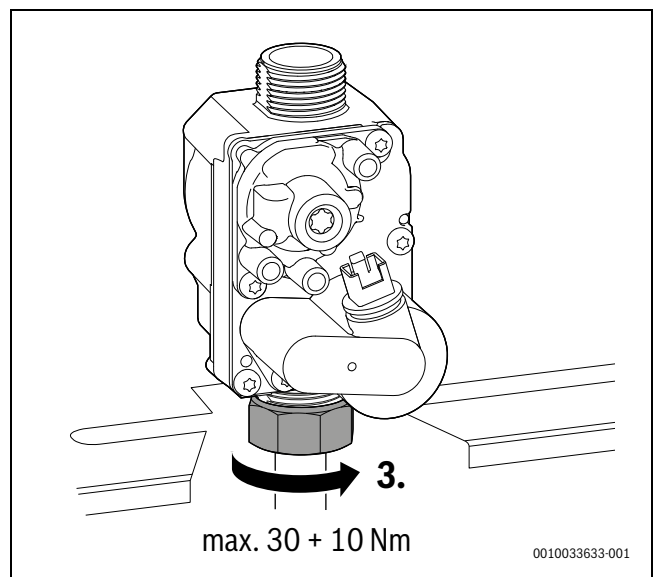
Bild 57 Anzugsdrehmoment beachten
