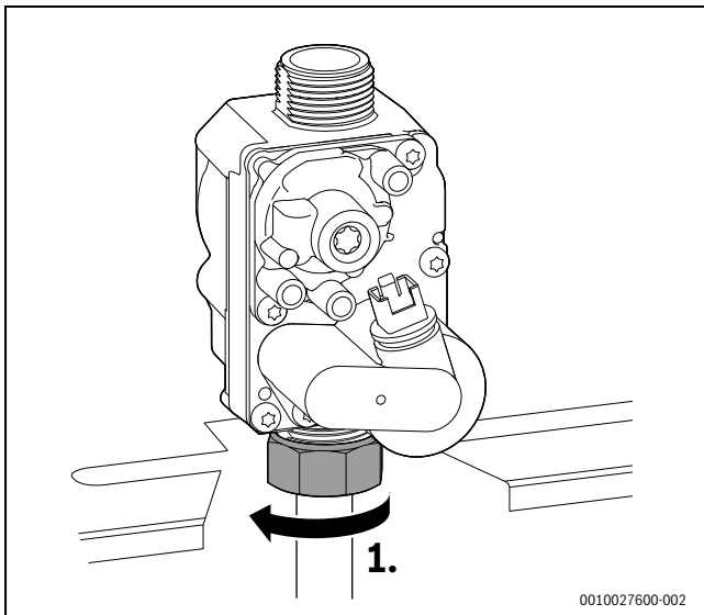
Bild 54 Überwurfmutter lösen
