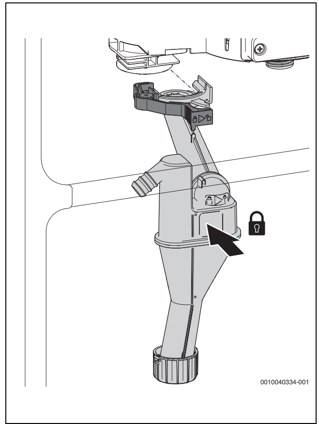
Bild 65 Kondensatsiphon einsetzen
