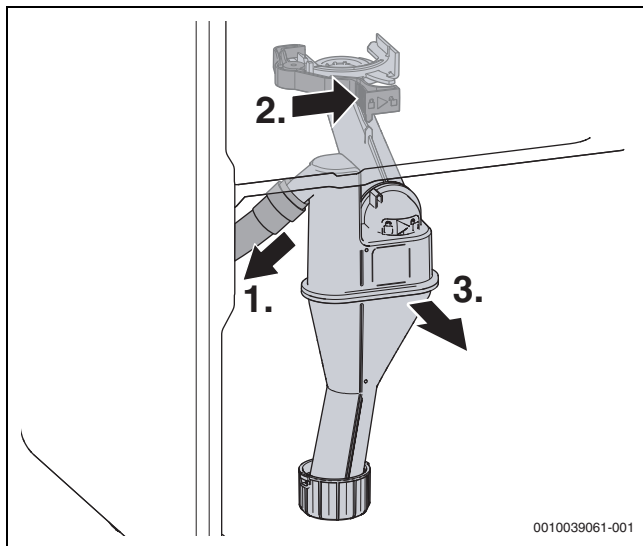
Bild 61 Kondensatsiphon ausbauen
