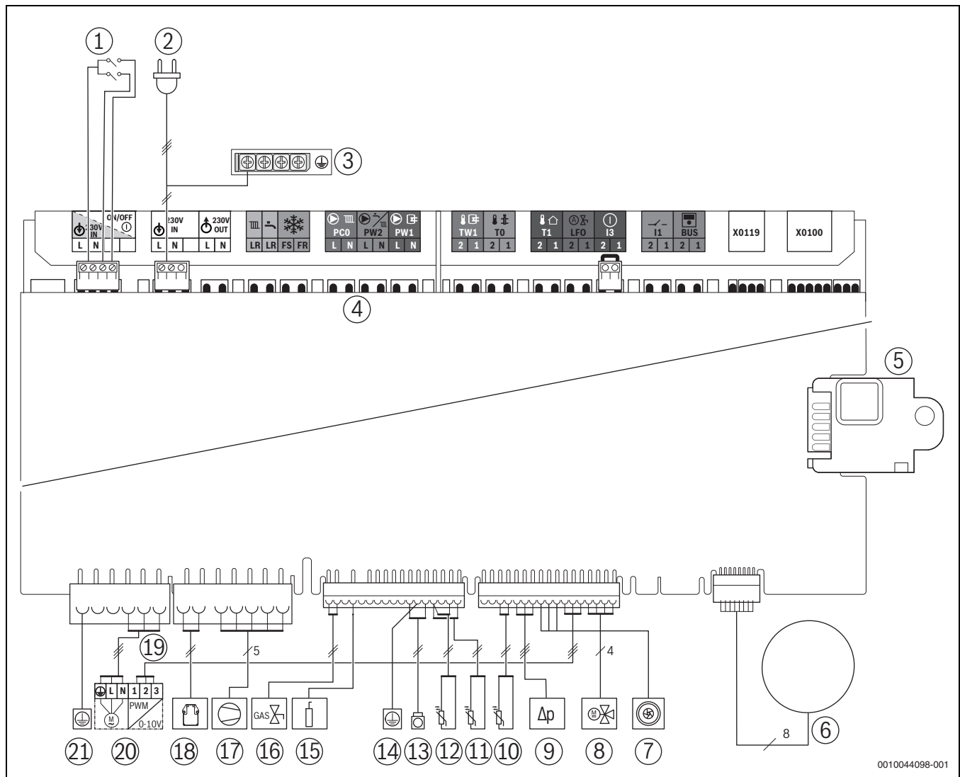
Bild 71 Elektrische Verdrahtung
