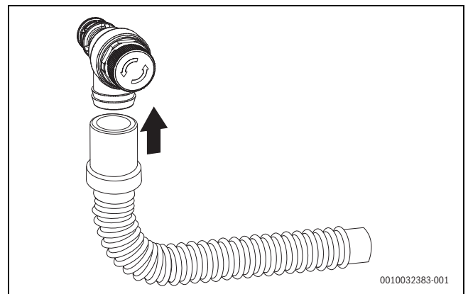
Bild 30 Schlauch am Sicherheitsventil (Heizung) montieren
