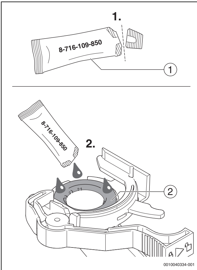
Bild 64 Dichtung fetten
