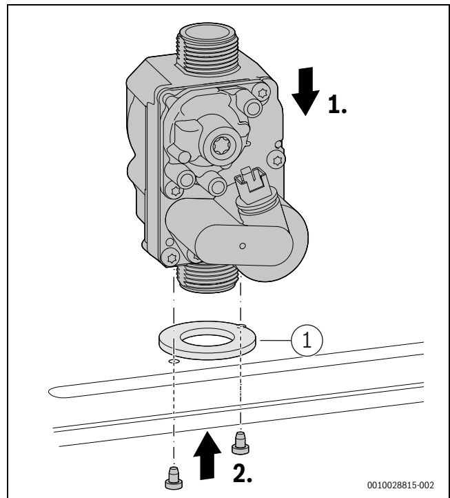
Bild 56 Gasarmatur einbauen
