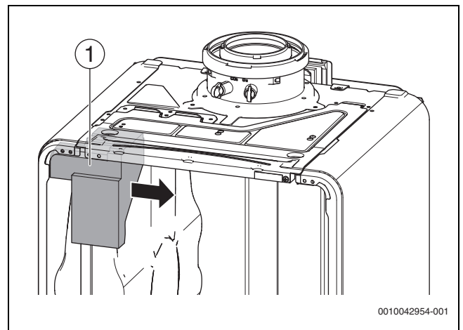
Bild 29 Stützschaum entfernen
