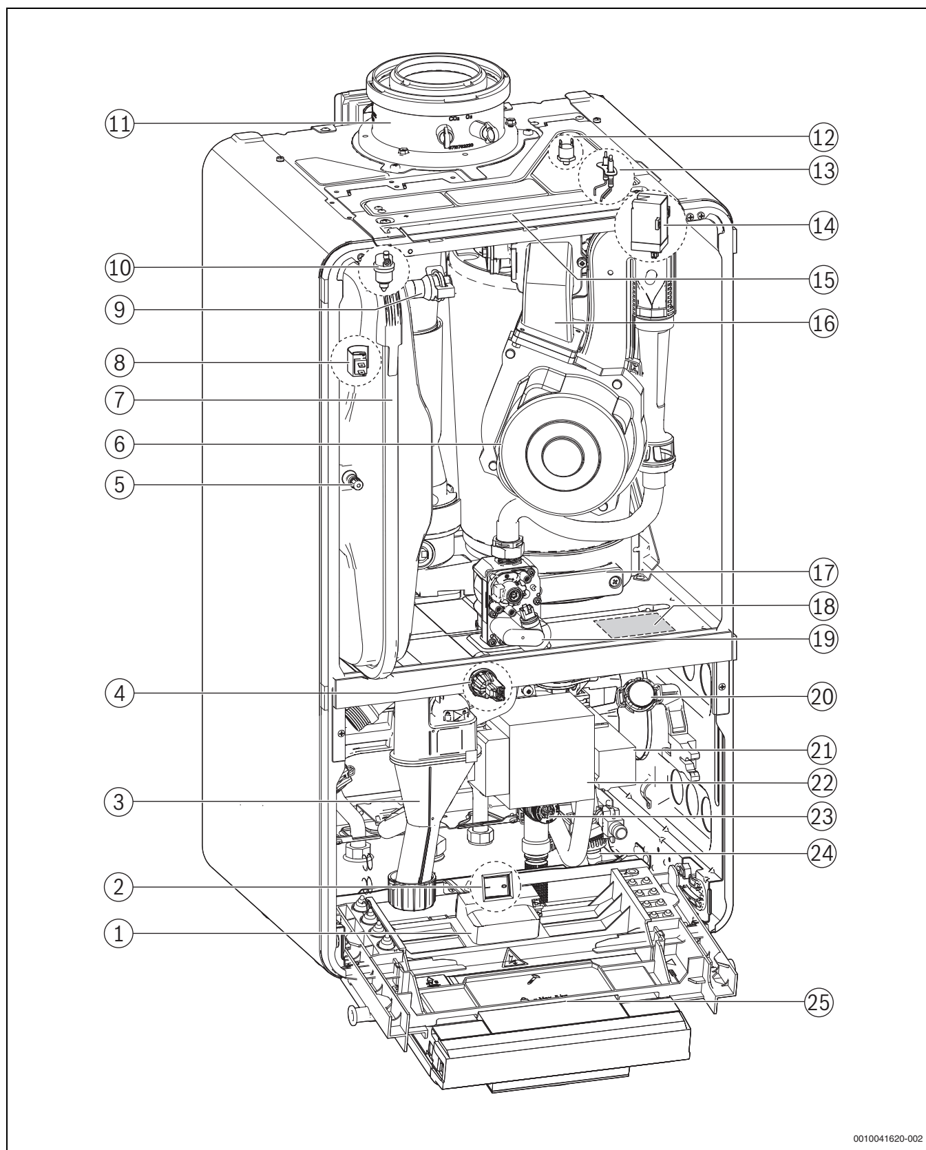
Bild 7 Produktübersicht
