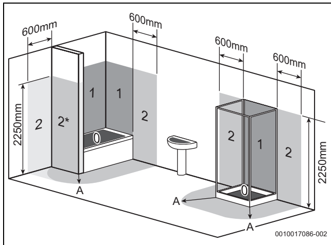
Bild 27 Schutzbereiche (Beispieldarstellung)
