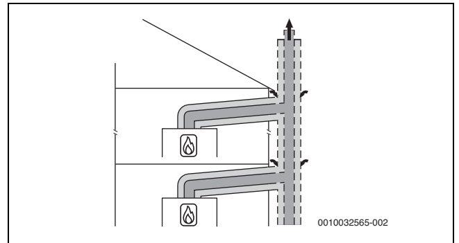
Bild 22 Mehrfachbelegung nach C (12)3x mit konzentrischer Luft-Abgas-Führung im Aufstellraum
