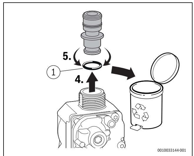
Bild 53 Gasdrossel abnehmen
