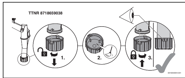
Bild 62 Schmutzfänger reinigen
