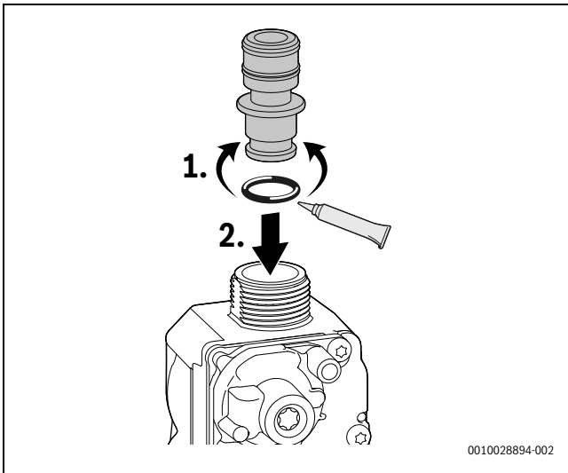
Bild 58 Gasdrossel einsetzen
