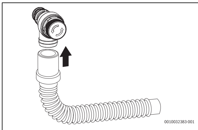
Fig. 30 Montage du tube sur la soupape de sécurité (chauffage)
