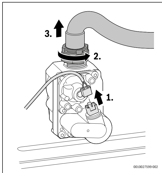
Fig. 52 Retrait du connecteur du bloc gaz et de l'écrou avec le tuyau du gaz
