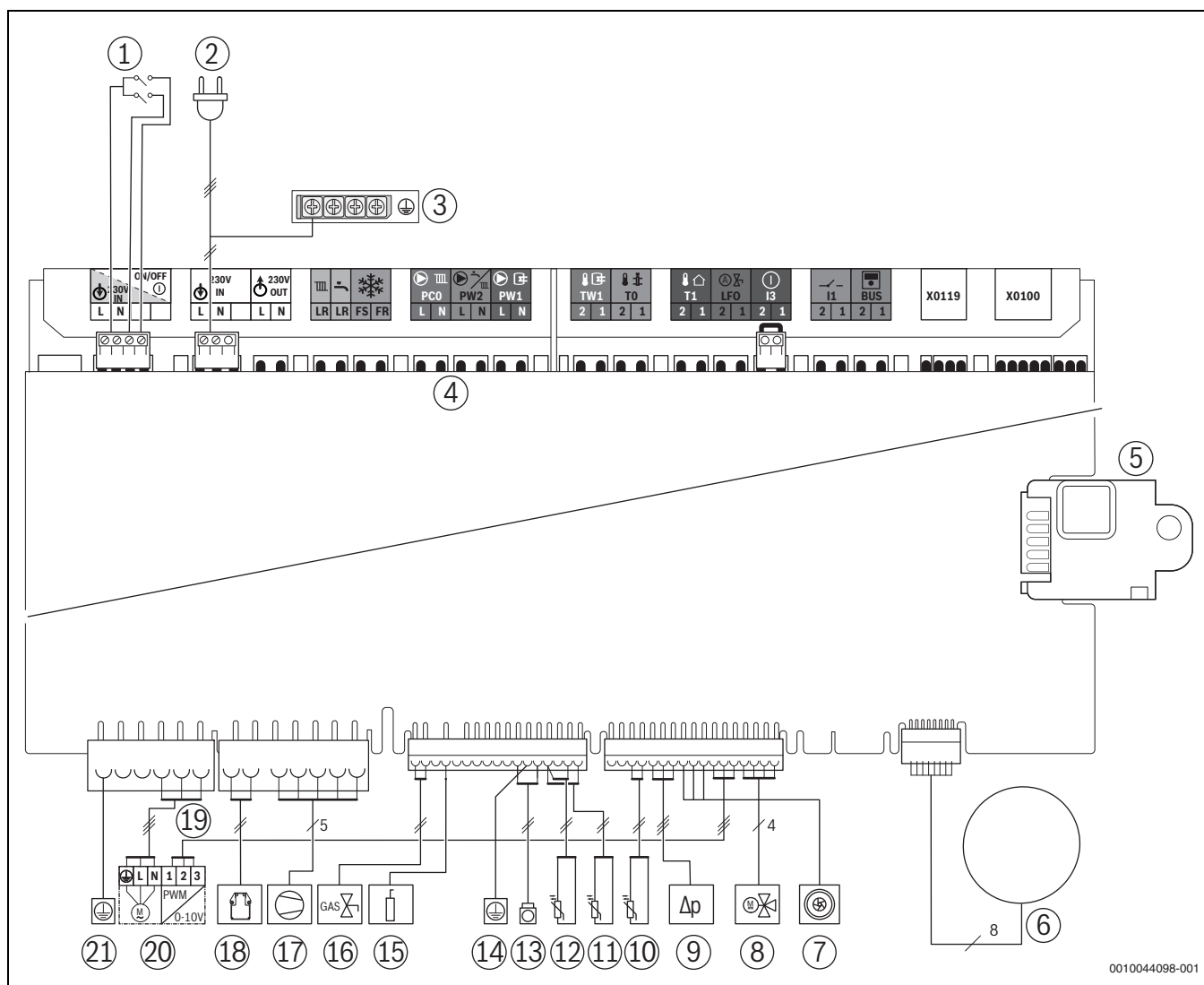
Fig. 71 Câblage électrique
