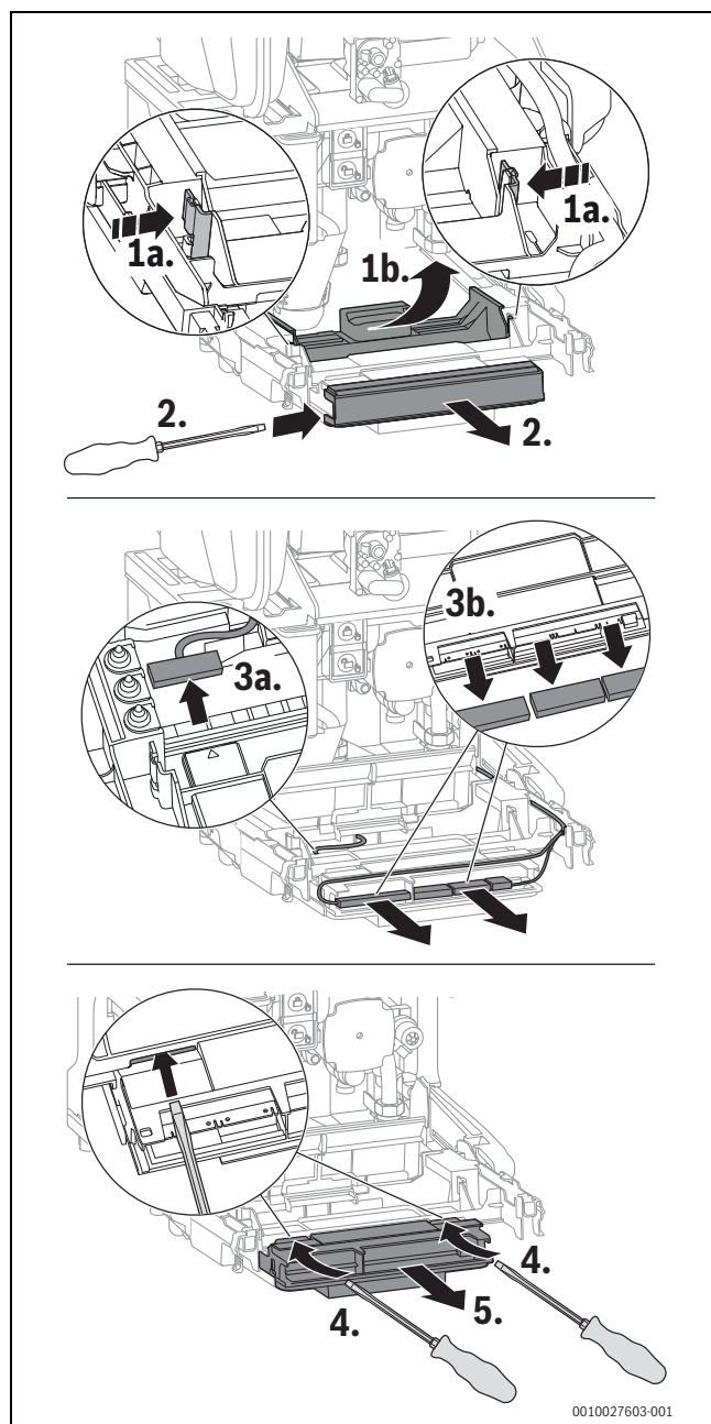
Fig. 60 Retirer l'appareil de commande
