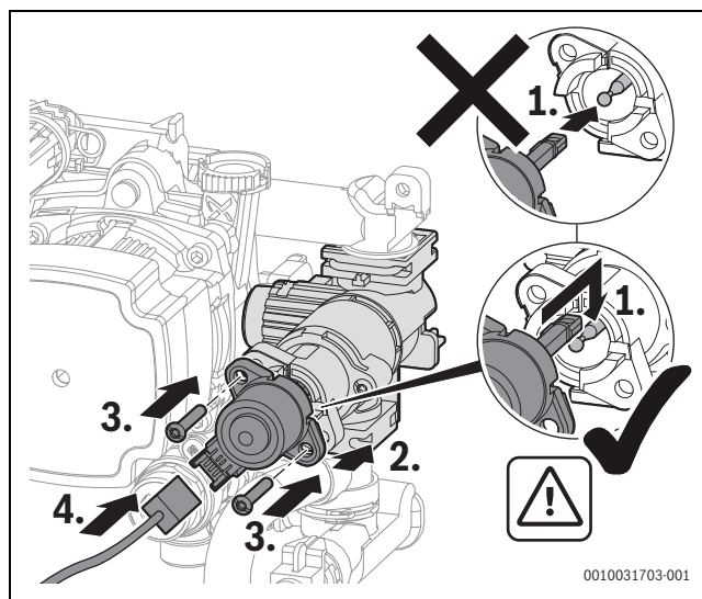
Fig. 69 Remonter le moteur au niveau de la vanne sélective (variante avec vis)
