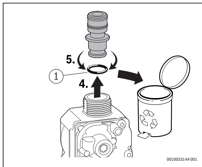
Fig. 53 Retrait de l'orifice
