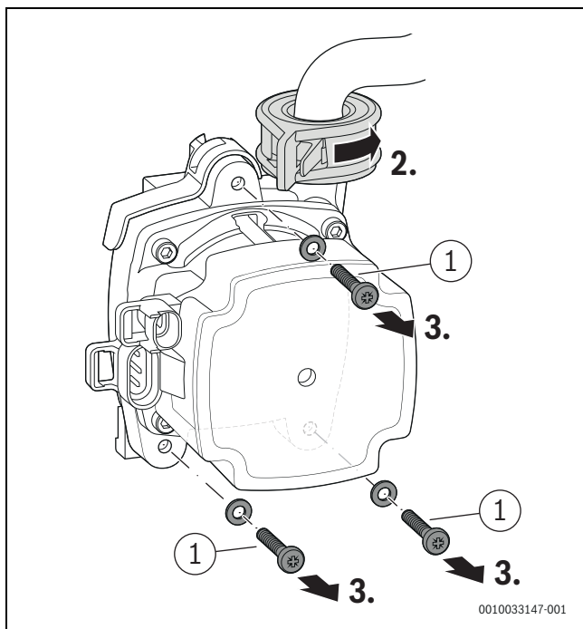
Fig. 49 Déverrouiller la pompe de chaudière et retirer les vis
