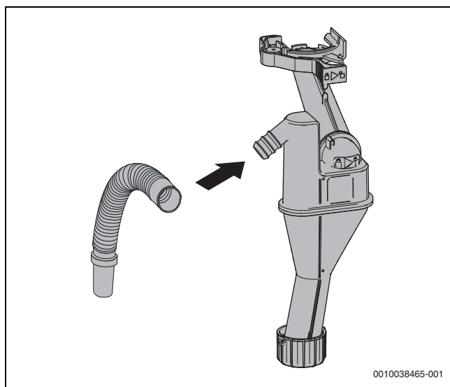
Fig. 31 Mettre l'évacuation des condensats sur le raccord
