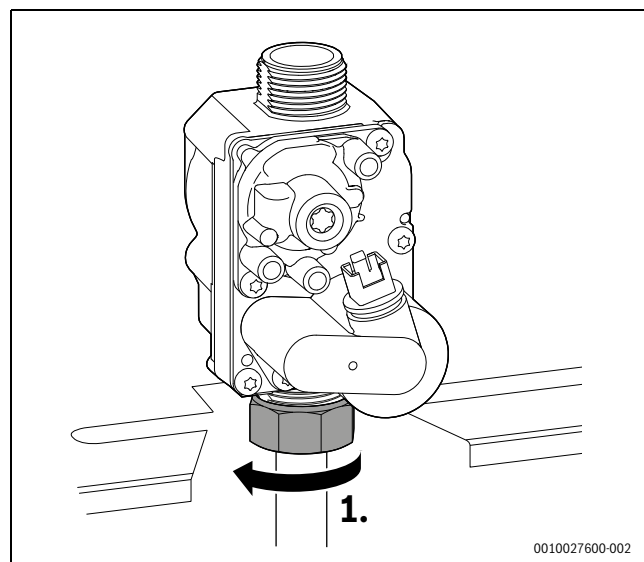
Fig. 54 Desserrage de l'écrou
