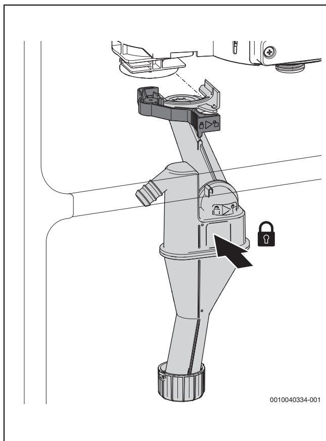
Fig. 65 Insertion du siphon de condensats
